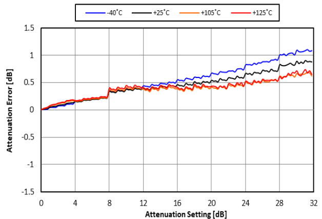
Figure 50. ATT Error vs Temp. @ 3500MHz
